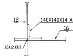
Ⓐ DET.
